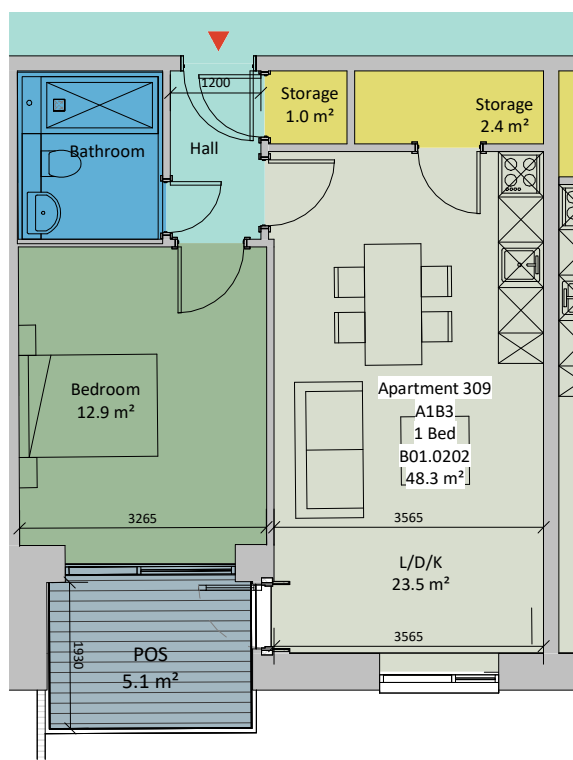
2 AT-A1B3 1 : 100
