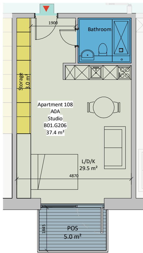
1 AT-A0A 1 : 100
