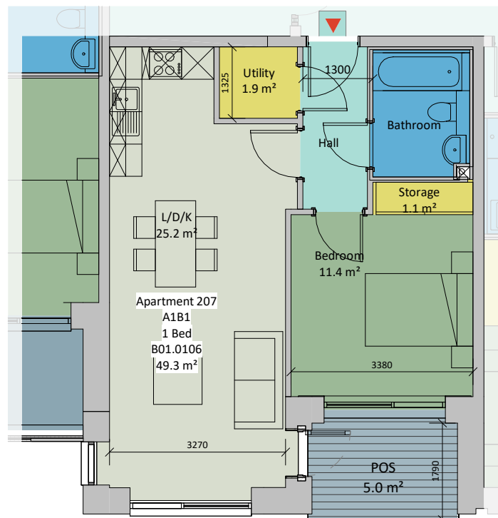
4 AT-A1B1 1 : 100
