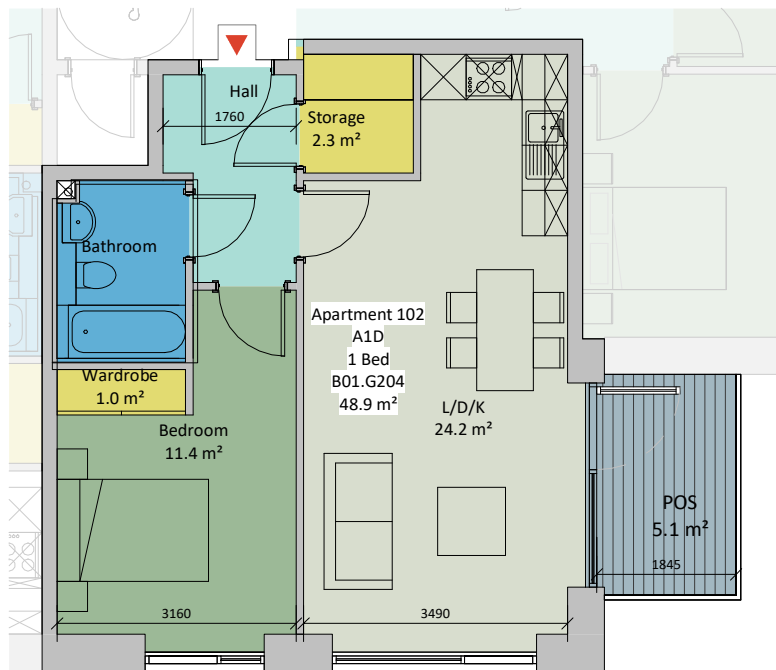
6 AT-A1D 1 : 100
