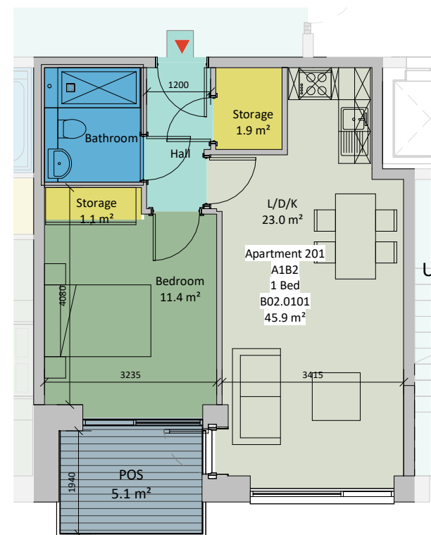
5 AT-A1B2 1 : 100
