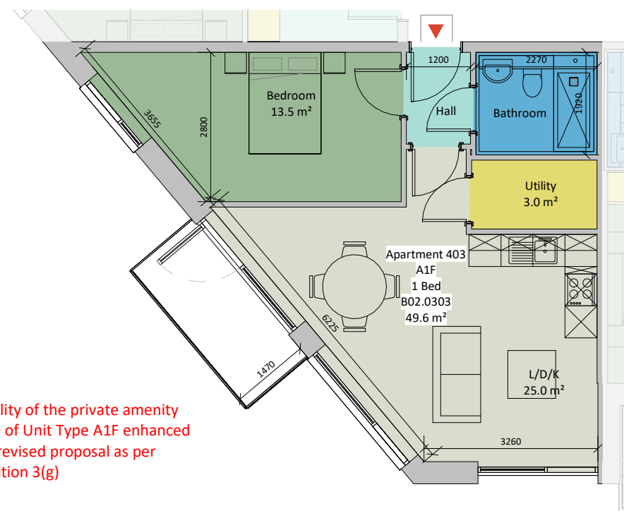
12 AT-A1F 1 : 100
