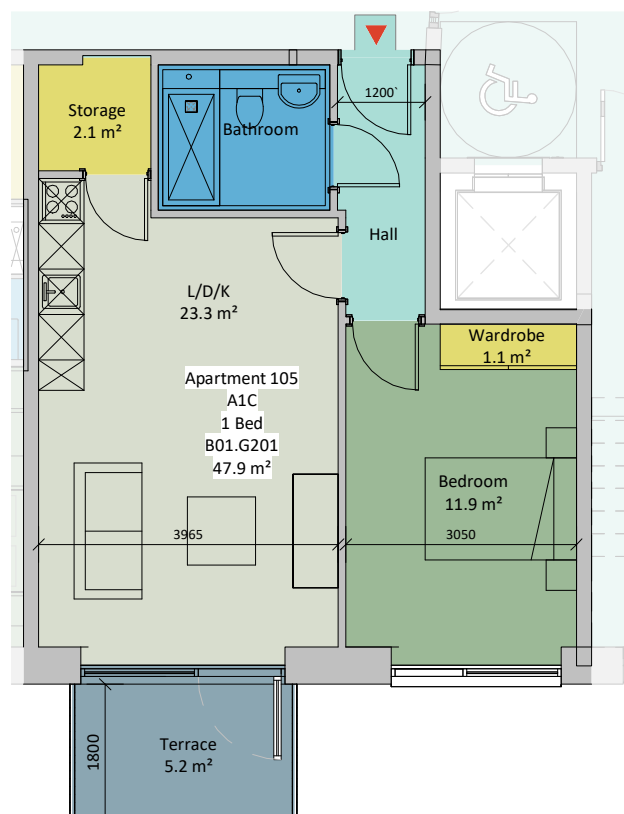
9 AT-A1C 1 : 100
