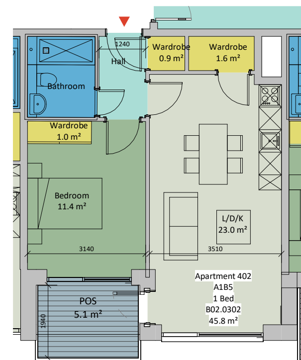
10 AT-A1B5 1 : 100
