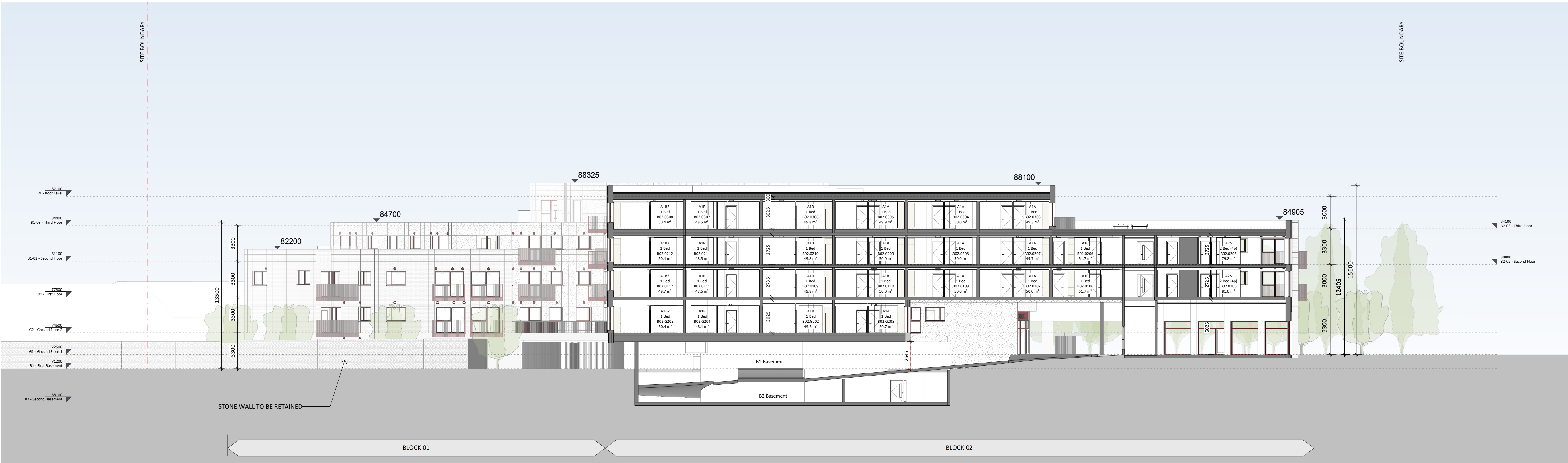
④ Section 4 - Block 02 Long Section 1 : 200
