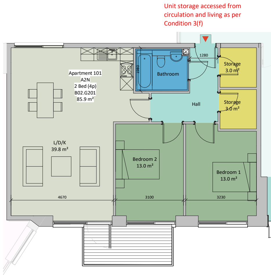
⑥ AT-A2N 1 : 100
