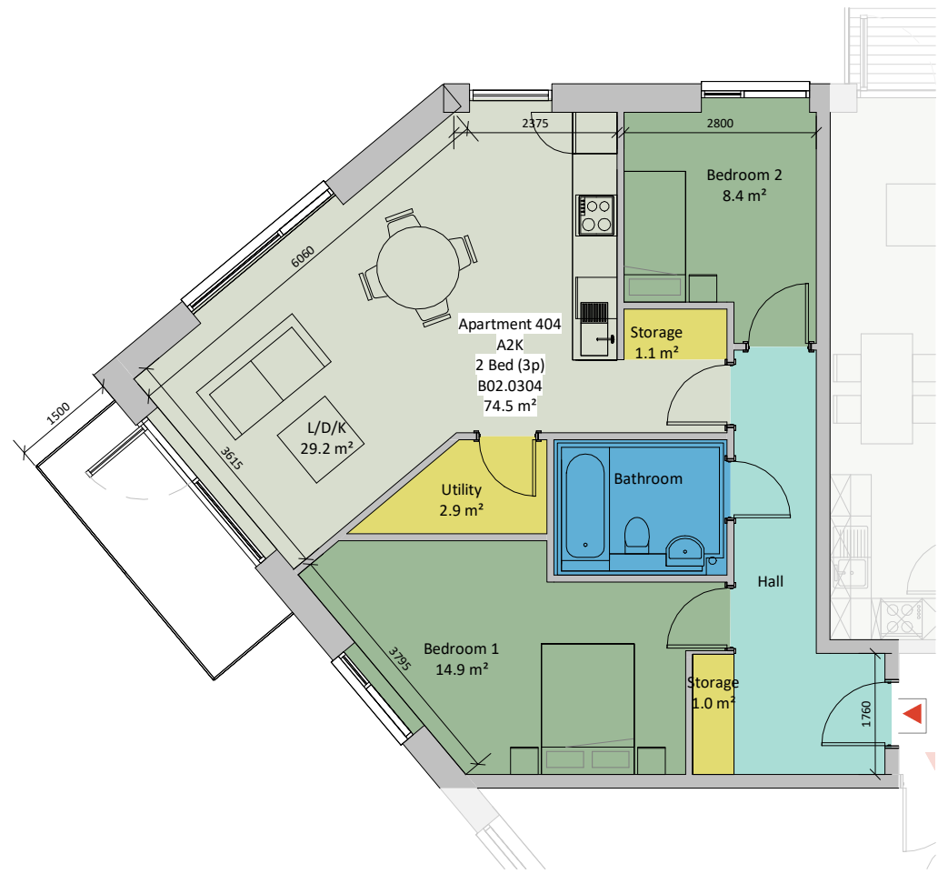
④ AT-A2K 1 : 100
