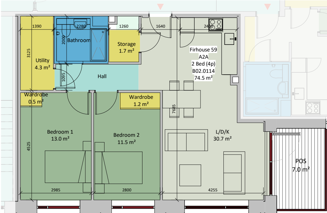
① AT-A2A 1:100
