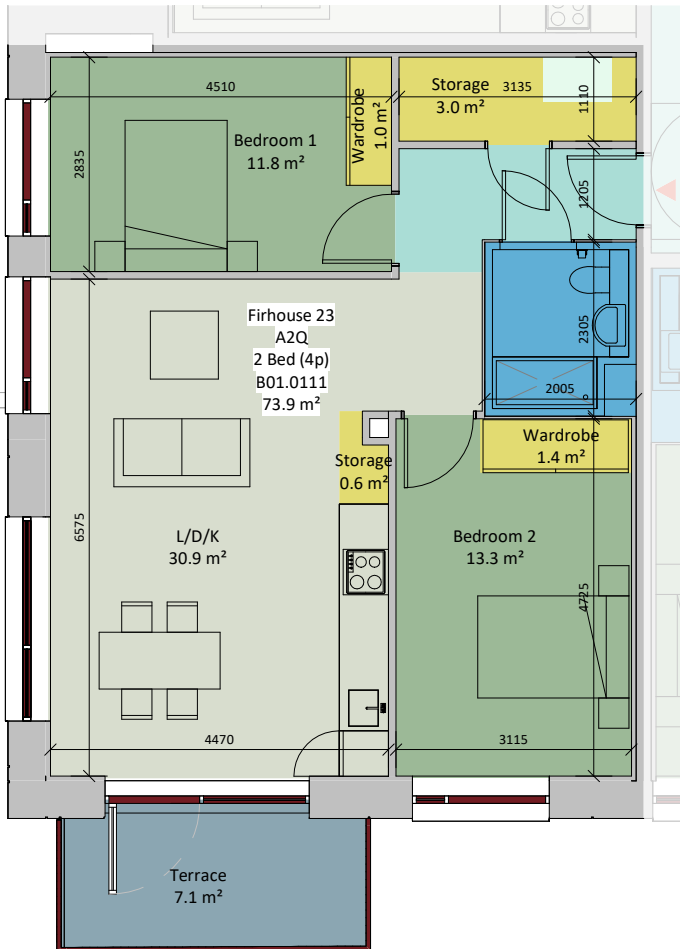
⑰ AT-A2Q 1:100
