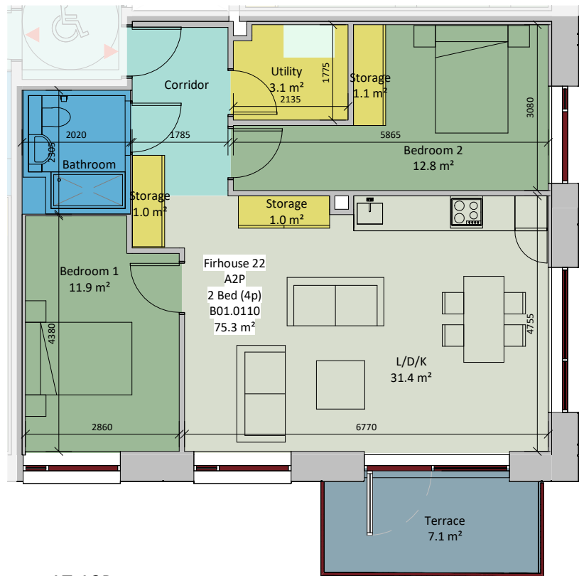
⑯ AT-A2P 1:100
