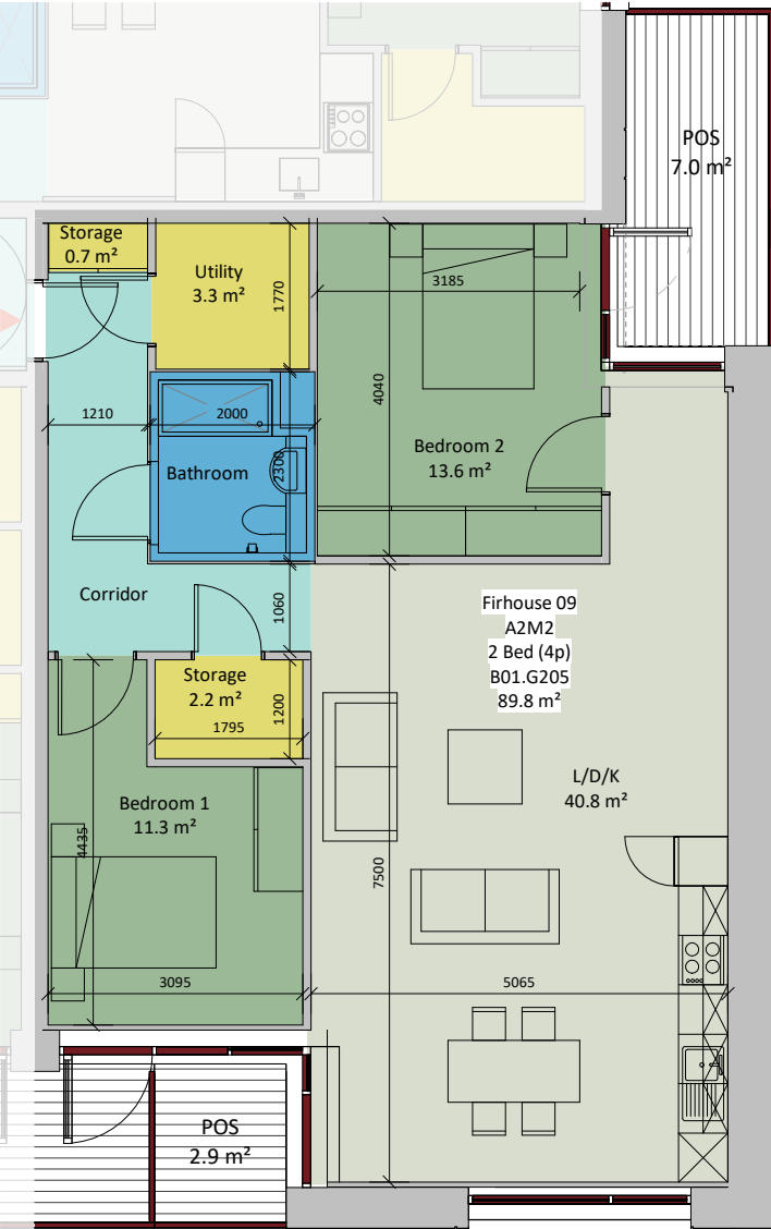
⑬ AT-A2M2 1:100
