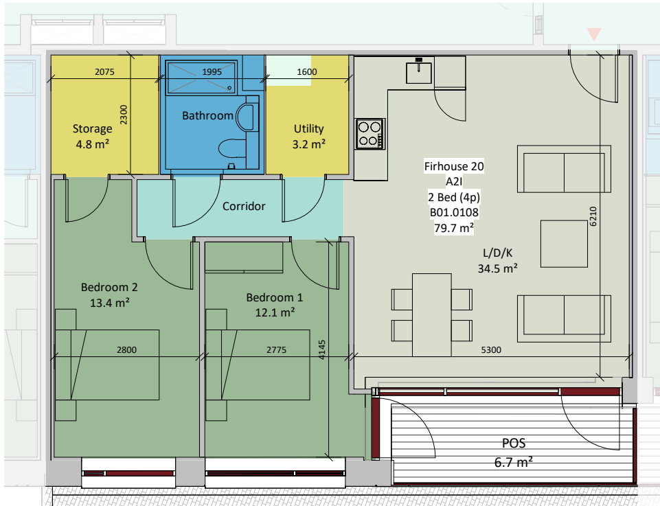
⑩ AT-A2I 1:100
