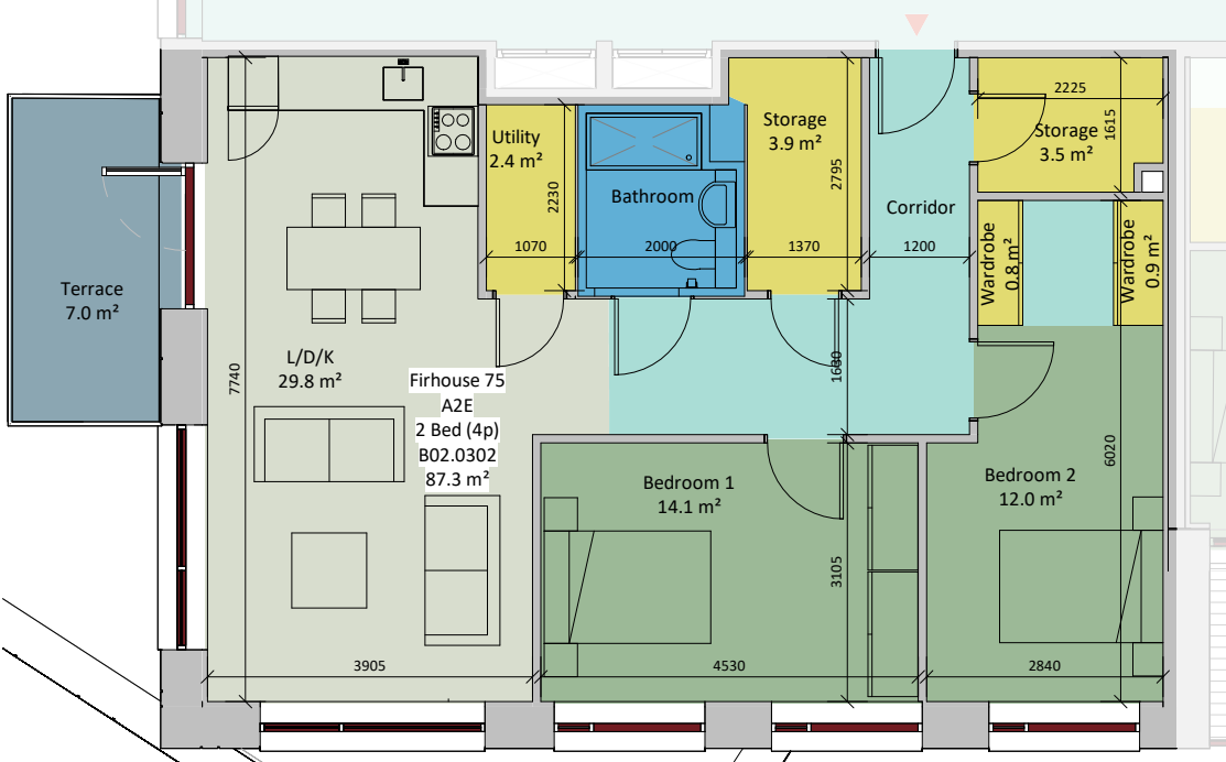
⑥ AT-A2E 1:100
