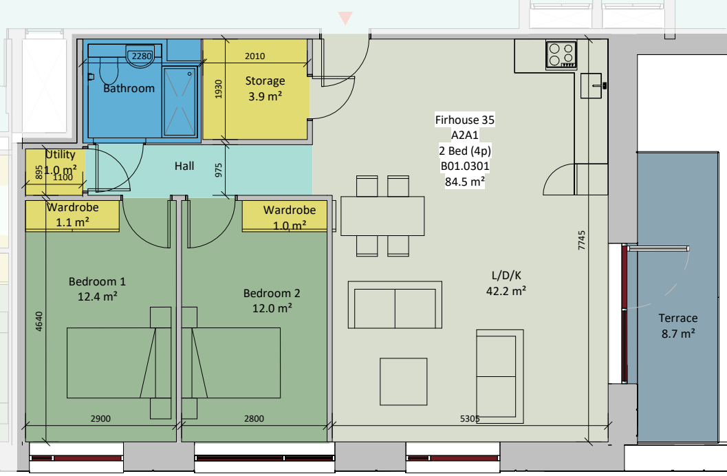
② AT-A2A1 1:100
