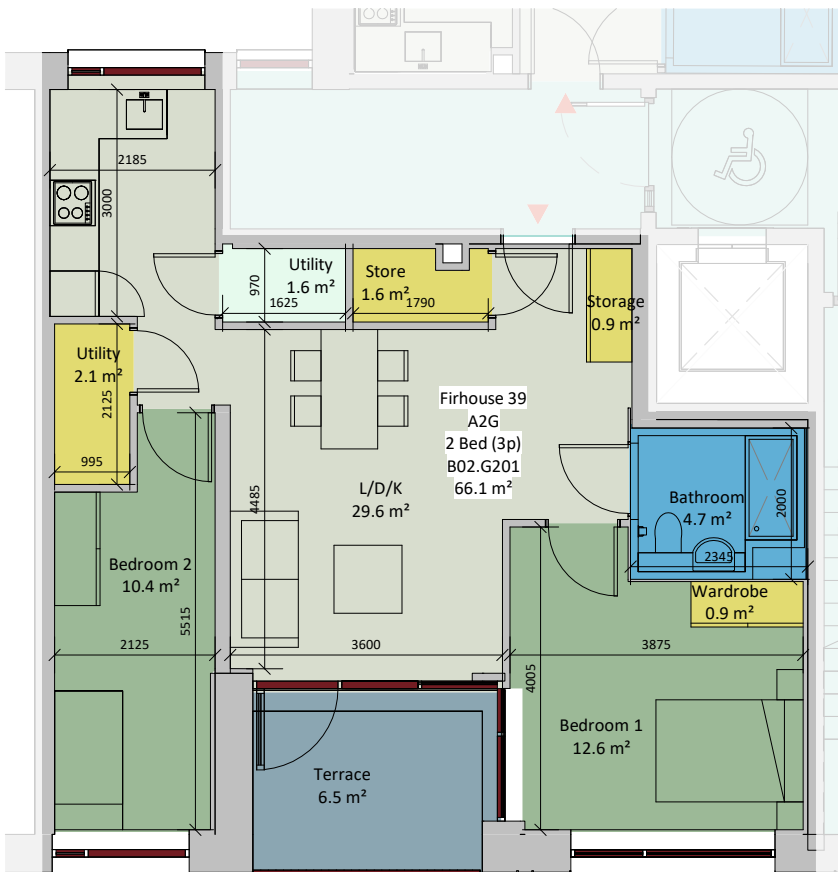
⑧ AT-A2G 1:100
