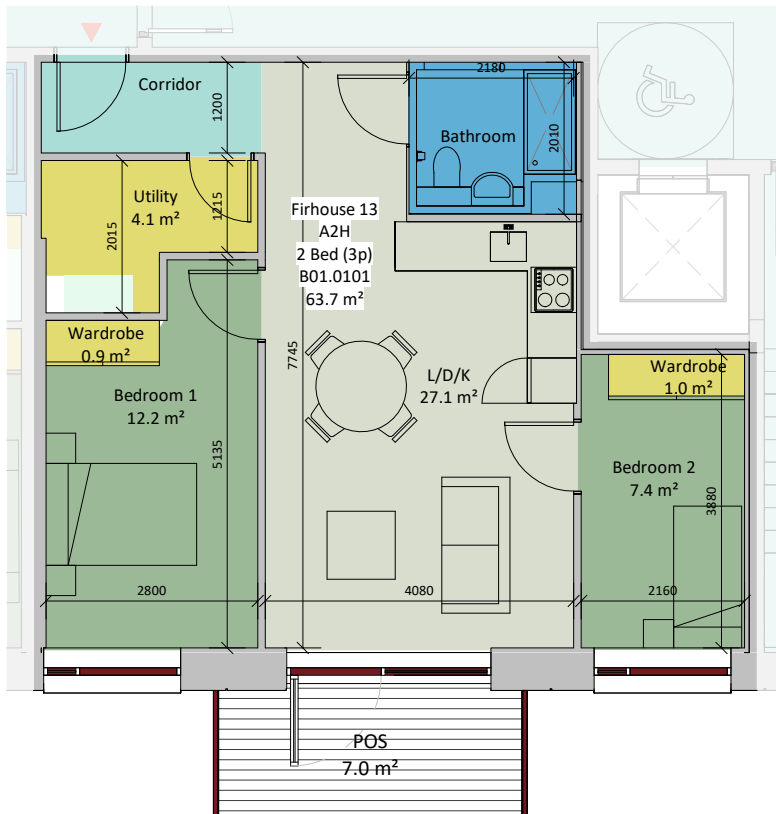
⑨ AT-A2H 1:100
